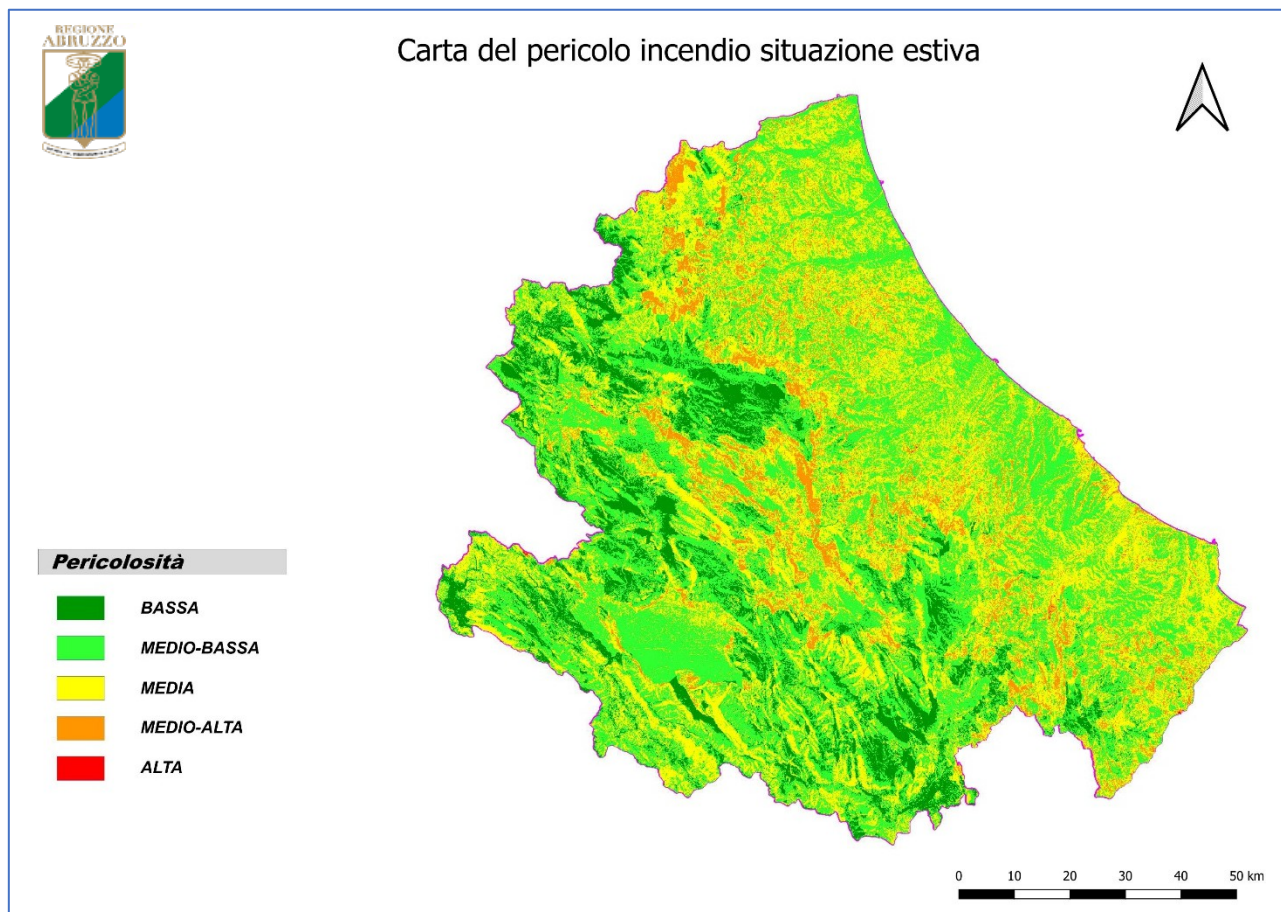
Fig. 4-15 - Carta della pericolosità situazione estiva
